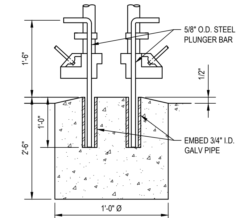
GATE PLUNGER BAR
